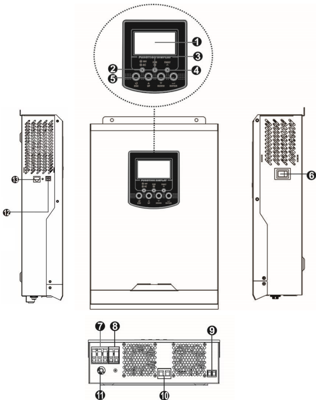
Рисунок 5. Инвертор SMARTWATT ECO 5K 48V 50A PWM.
