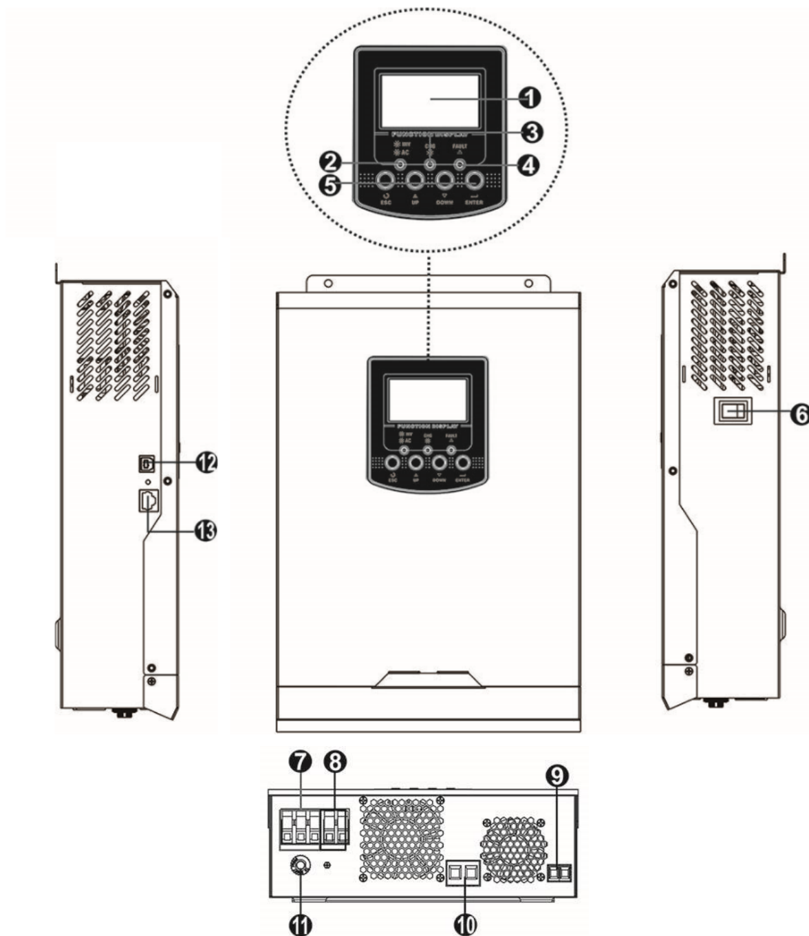
Рисунок 4. Инверторы SMARTWATT ECO 3K 24V PWM и SMARTWATT ECO 3K 24V MPPT
