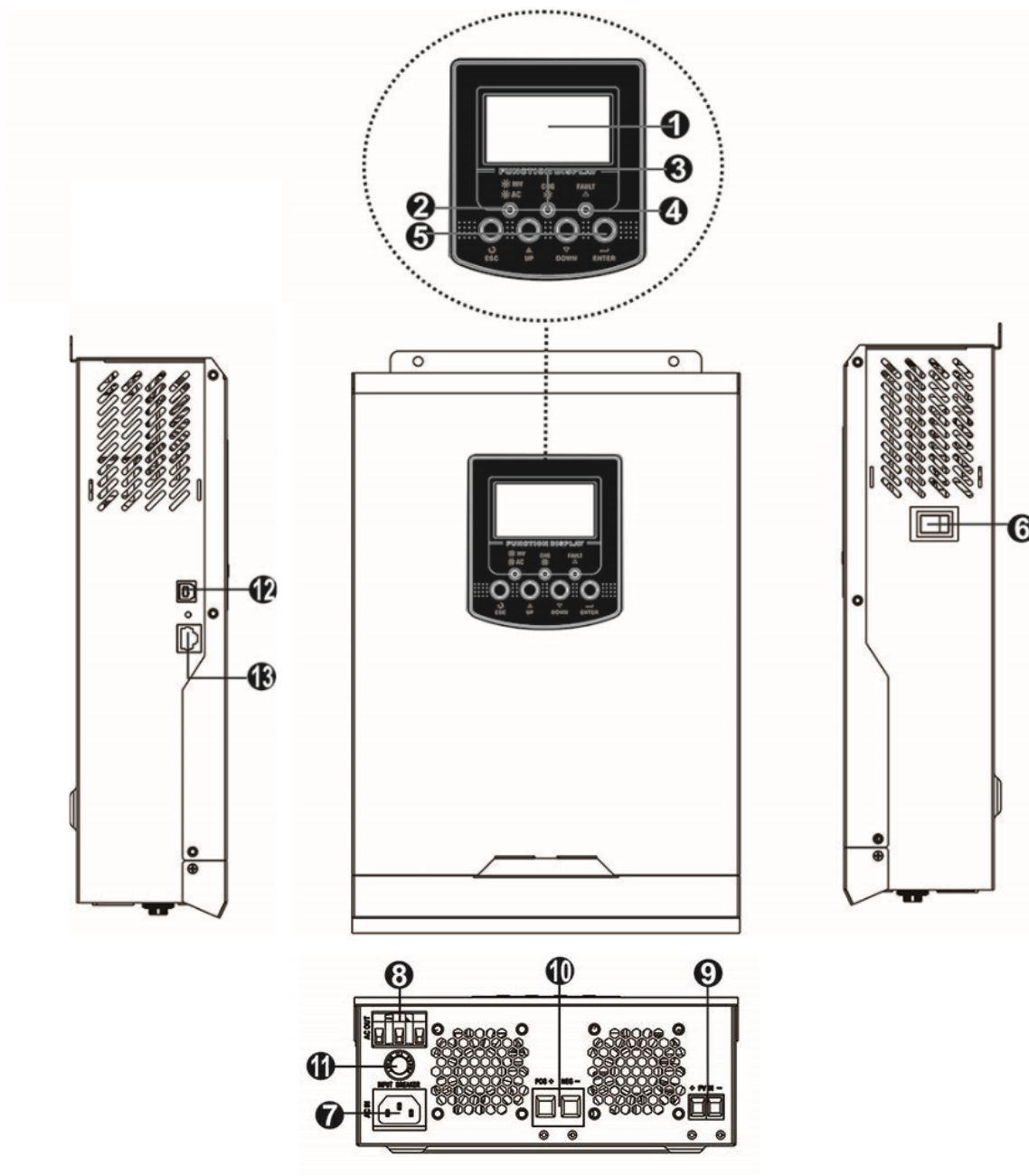
Рисунок 2. Инвертор SMARTWATT ECO 1K 12V PWM.
