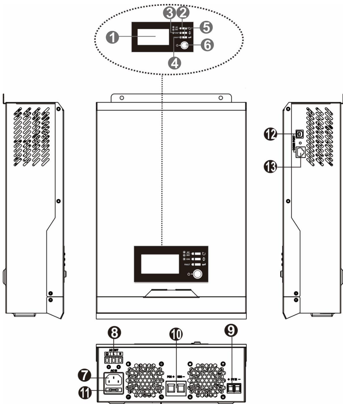
Рисунок 3 Инвертор SMARTWATT ECO 1K 12V MPPT.
